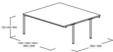
Bench Twin Baukasten - Anfangsmodul
