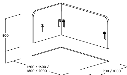
Hauteur fixe – Paroi latérale gauche ou droite (400 / 500 / 600) dessus plan de travail
