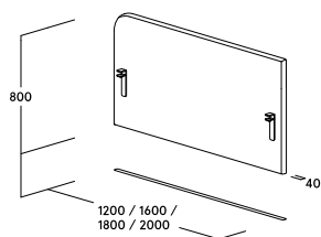
Hauteur fixe – Rayon à gauche ou à droite (400 / 500 / 600) dessus plan de travail
