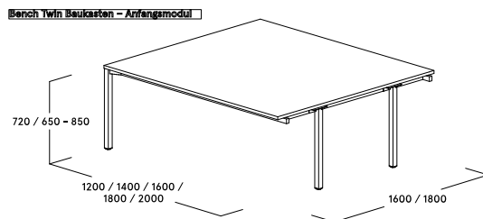
Bench Twin Baukasten - Anfangsmodul
