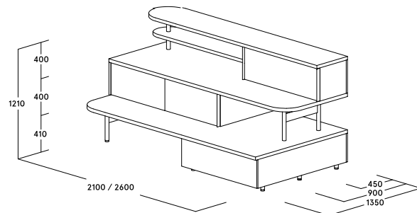
arena Grundmodul (freistehend)
