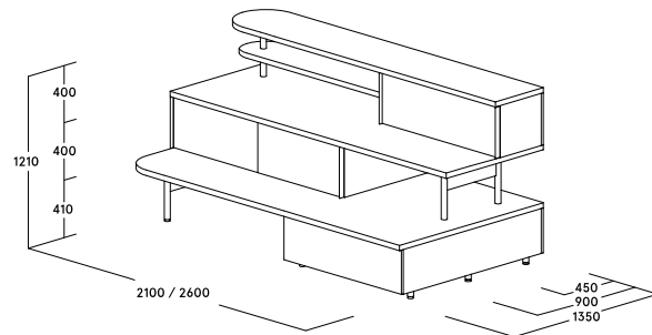
arena Grundmodul vorbereitet für Anbau rechts
